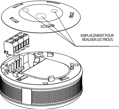
Schéma 2 – Montage des raccordements à la source d'alimentation et au système d'alarme.
