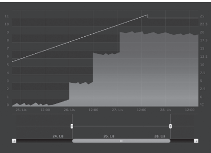
Figure 3. Visualisation des données de la boîte noire du Fibaro Smoke Sensor.
