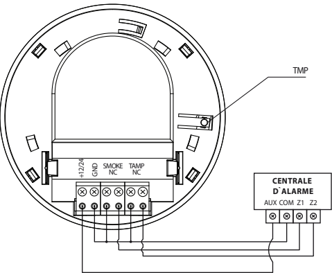
Schéma 4 – connexion du Fibaro Smoke Sensor au système d'alarme.
