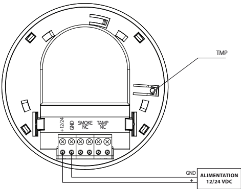
Schéma 3 – raccordement à la source d'alimentation continue.
